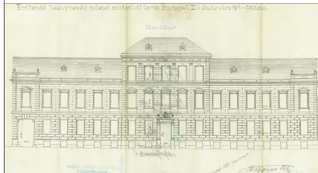
A Jó Pásztor Rendház második homlokzatterve, 1891, tervező–kivitelező Hofhauser Elek BFL XV.17.d 329.17345/1
