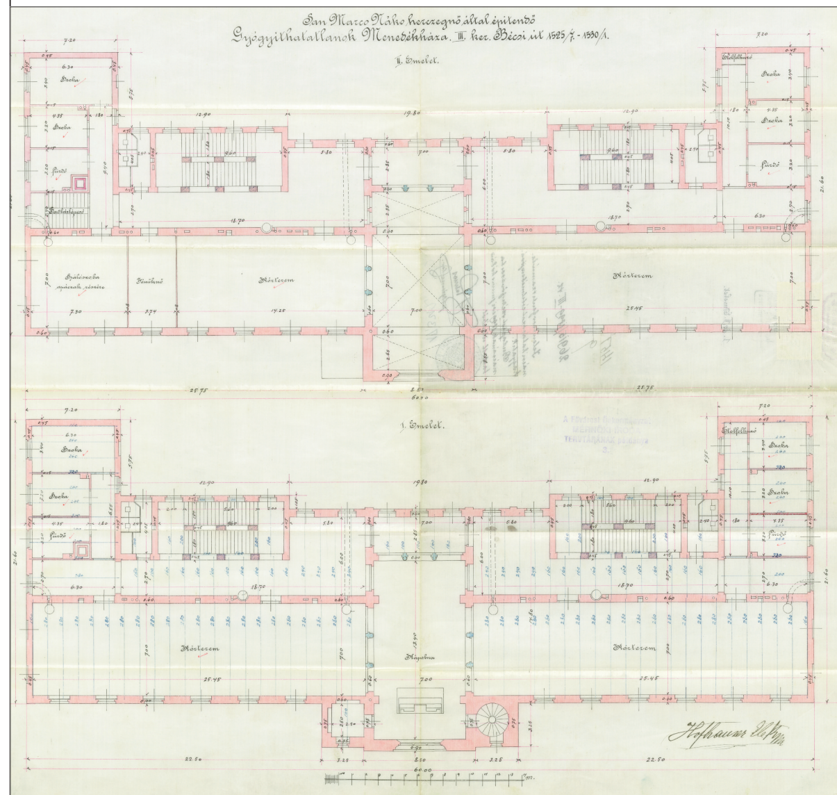
Az Irgalom Háza emeleti szintjeinek alaprajza (1900, Hofhauser Elek) BFL XV.17.d. 329 17321
