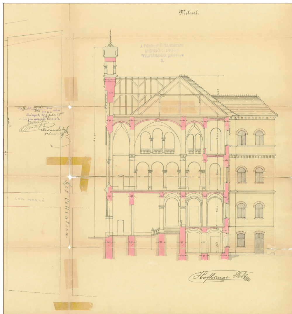
Az Irgalom Háza keresztmetszete (1900, Hofhauser Elek) BFL XV.17.d. 329 17321
